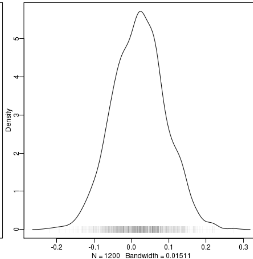
\beta の事後確率密度の推定
